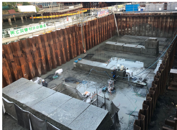
橋撤去状況写真 (イメージ)
