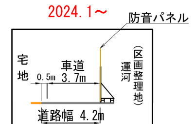
A-A断面図
