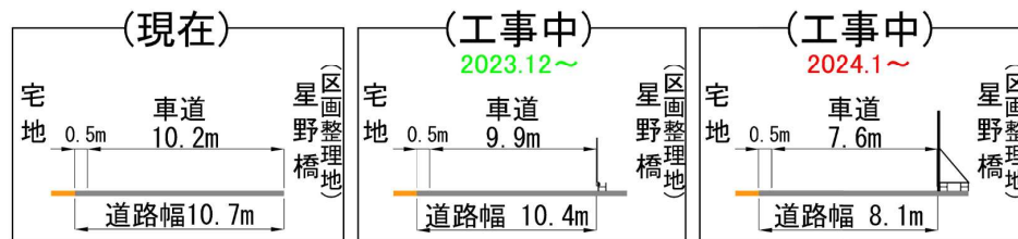
A-A 断面
