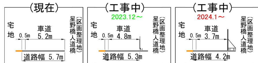
B-B 断面
